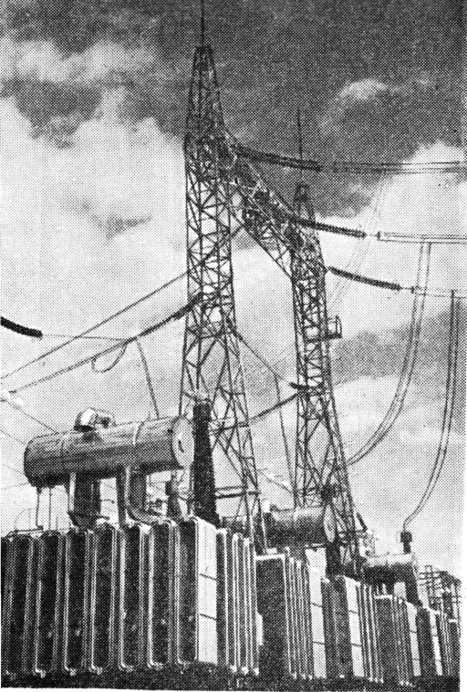
Новая трансформаторная группа.
